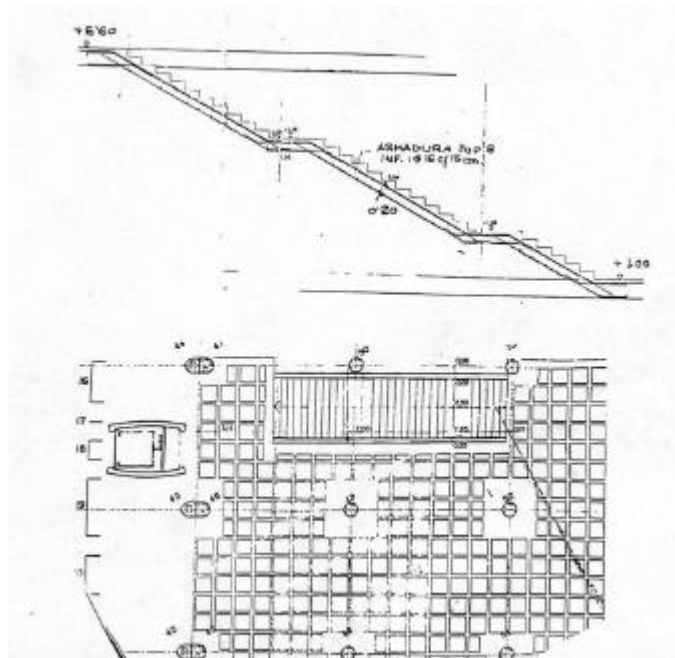
Figura 2. Planta y alzado de la losa de escalera.
