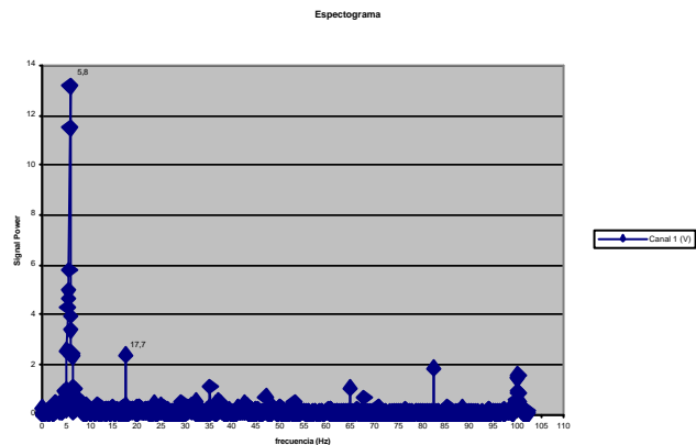
Figura 6. Espectrograma de frecuencias tramo central
