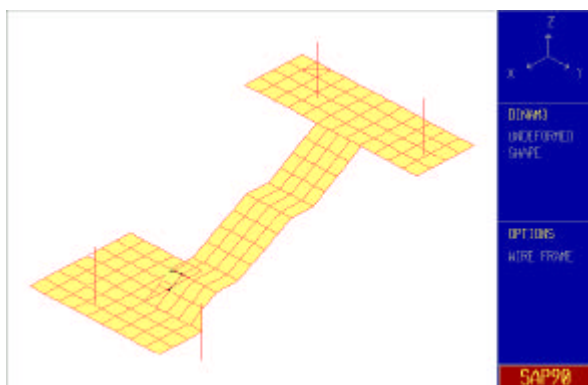
Figura 3. Modelo tridimensional de elementos finitos
